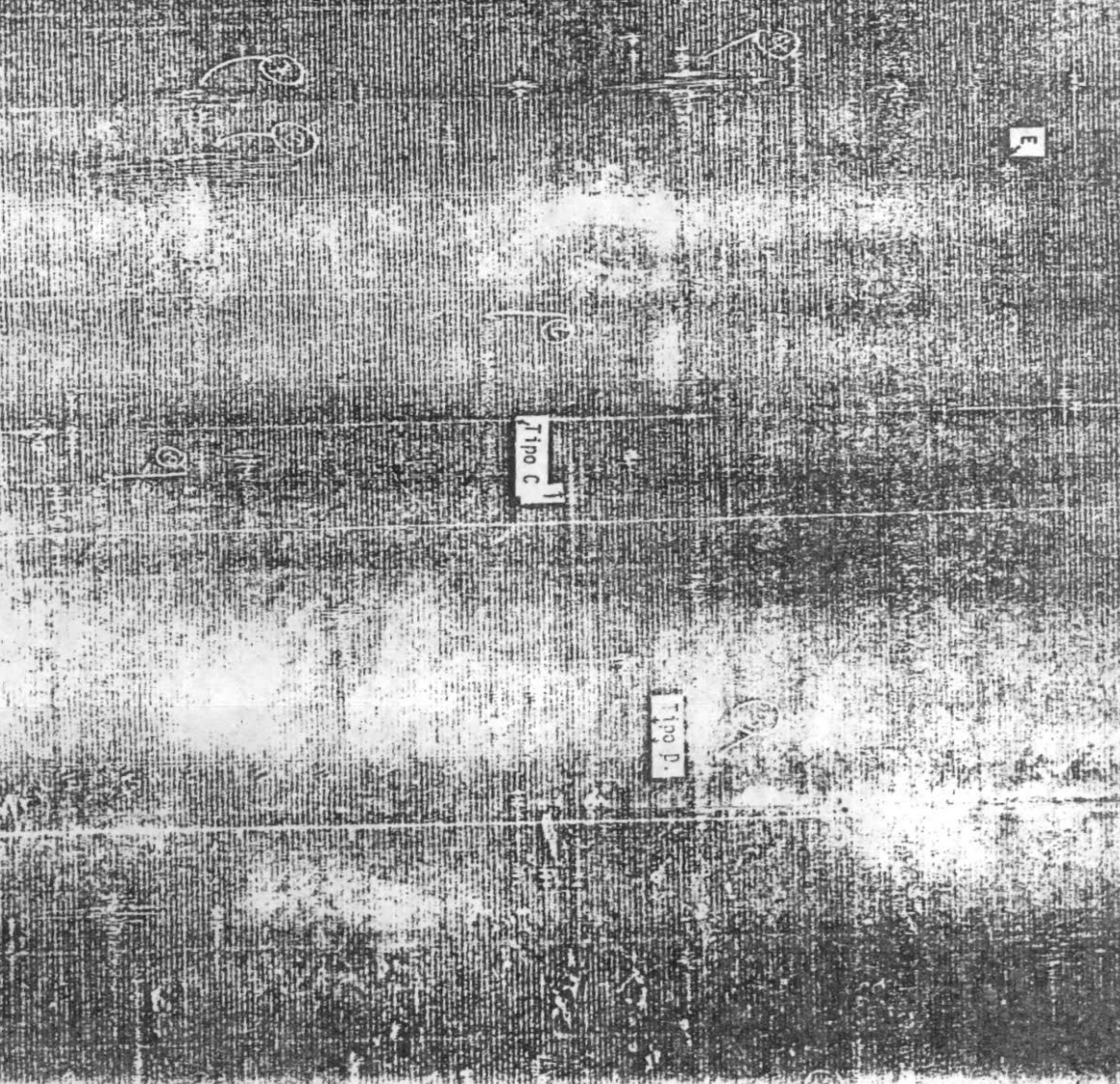
FIGURA 16: TREMORES DEL VOLCAN NEVADO DEL RUIZ Obsérvese los tremores de alta frecuencia (Tipo C) y los de baja frecuencia (Tipo D) y los espasmos (E). Nótese la dificultad para precisar el momento de inicio y finalización del tremor. Sismograma Estación REFUGIO 1, 20-21 de Julio/85.
