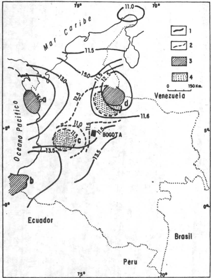
Mapa de energía sísmica promedio liberada anualmente. 1-H 70Km. 2-H 70 Km. 3-4.Zonas de alta sísmicidad. a) Choco. b). Nariño. c)Caldas. d) Santander.
