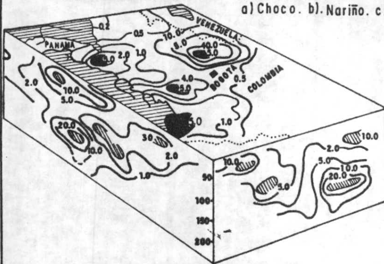
Densidad de hipocentros y distribución de focos sísmicos con la profundidad.
