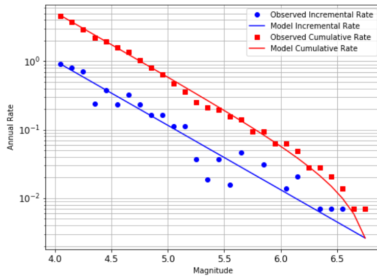
Figura D.6. Distribución de magnitud y frecuencia, fuente Andina (c05)
