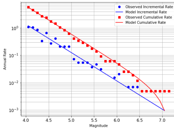
Figura D.2. Distribución de magnitud y frecuencia, fuente Pacífica (c01)
