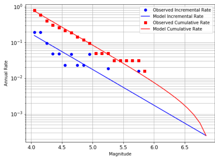
Figura D.9. Distribución de magnitud y frecuencia, fuente Panamá (p00)
