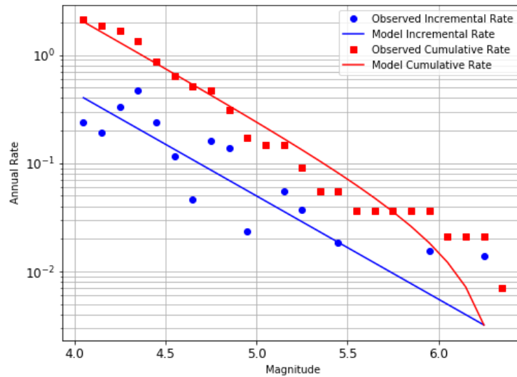
Figura D.1. Distribución de magnitud y frecuencia, fuente Guajira - Paraganá (c00)
