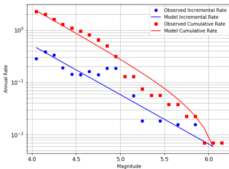
Figura D.3. Distribución de magnitud y frecuencia, fuente Nororiental (c02)
