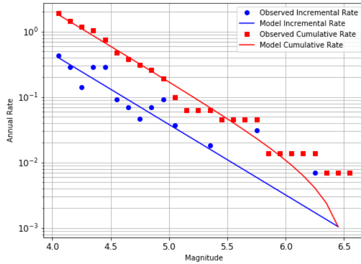
Figura D.7. Distribución de magnitud y frecuencia, fuente Caribe (c06)
