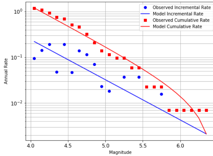
Figura D.5. Distribución de magnitud y frecuencia, fuente Oca - Falcón (c04)
