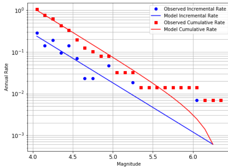
Figura D.8. Distribución de magnitud y frecuencia, fuente Cratón (c07)
