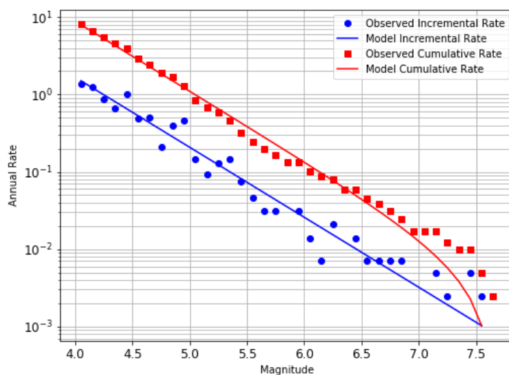
Figura D.4. Distribución de magnitud y frecuencia, fuente Piedemonte oriental (c03)
